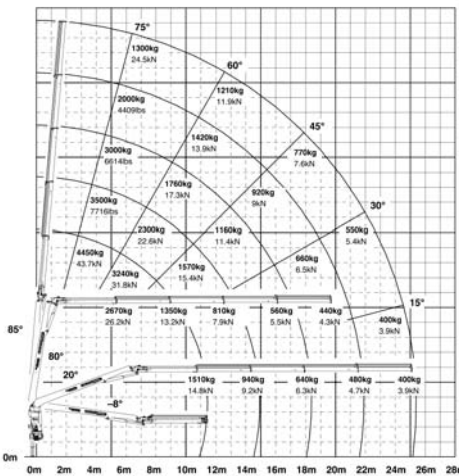
PK 25001 EL Performance C
