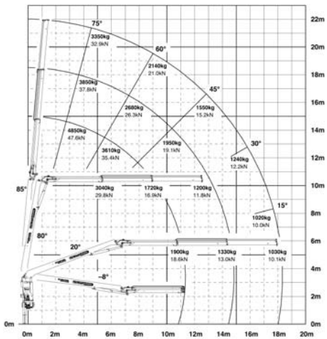
PK 25001 EL Performance A
