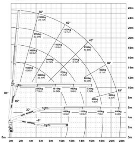
PK 25001 EL Performance B
